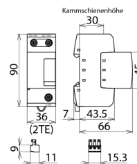
Maßbild DSE M 1 60 FM
