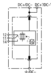
Prinzipialschaltbild DSE M 1 220 FM
