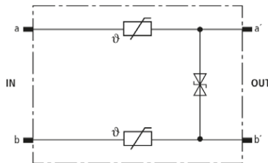
Prinzipschaltbild DRL PD 180
