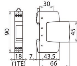
Maßbild DR M 2P 255
