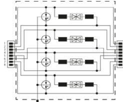
Prinzip Schaltbild DPA M CAT6 RJ45S 48
