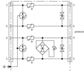
Prinzipschaltbild DLI TC 2 I
