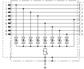
Prinzipschaltbild FS 9E HS 12
