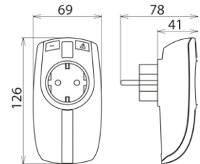
Maßbild DPRO 230
