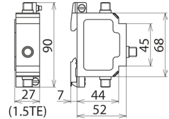
Maßbild DGA FF TV
