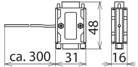
Maßbild FS 9E HS 12
