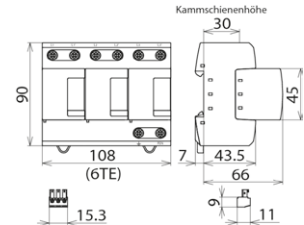
Maßbild DV M TNC 255 FM
