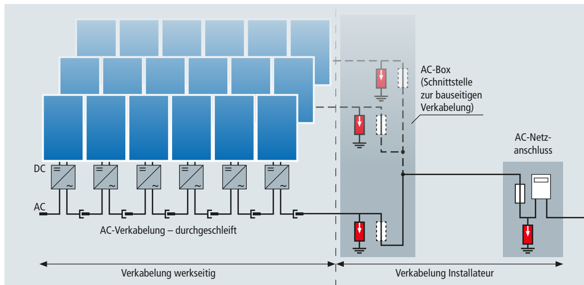
Bild 16 Beispiel: Gebäude ohne äußeren Blitzschutz; Überspannungsschutz für Modulwechselrichter befindet sich im Anschlussgehäuse der bauseitigen Verkabelung
