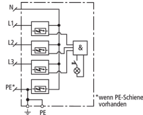
Prinzipialschaltbild DSH ZP B TT 255
