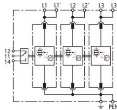
Prinzipialschaltbild DV M TNC 255 FM
