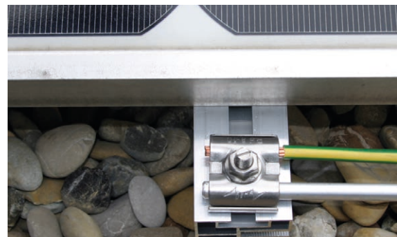
Bild 3 UNI-Erdungsklemme: Ein Edelstahl-Zwischenelement vermeidet Kontaktkorrosion. Dadurch werden langjährige sichere Verbindungen zwischen unterschiedlichen Leiterwerkstoffen geschaffen
