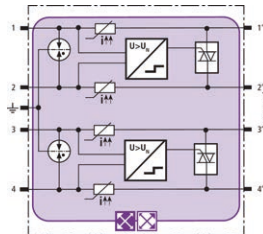
Principalschaltbild BXTU ML4 BD 0-180
