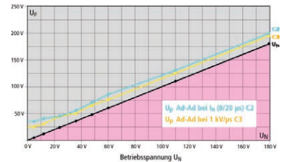
Schutzpegeldiagramm BXTU
