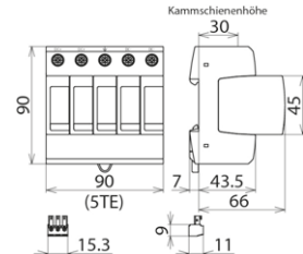
Maßbild DG M PV2 SCI 1000 FM
