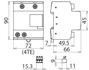
Maßbild DCB YPV SCI 1000 FM
