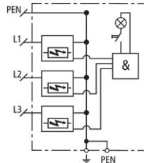
Principalschaltbild DSH ZP B TNC 255
