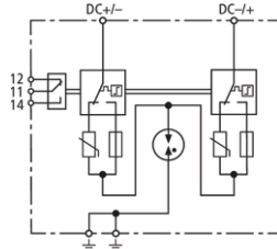
Prinzipialschaltbild DCB YPV SCI 1000 FM
