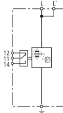
Prinzip Schaltbild DBM 1 760 FM
