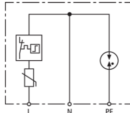
Prinzip Schaltbild DCOR L 2P 275
