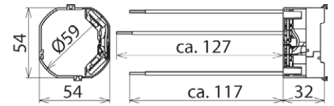
Maßbild STC 230
