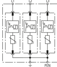
Prinzipschaltbild DG M WE 600
