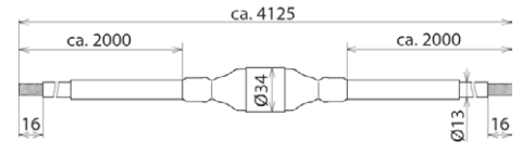
Maßbild EXFS 100 KU
