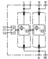
Prinzipialschaltbild DV M TN 255 FM
