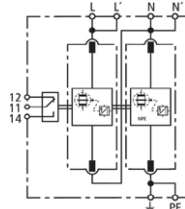
Principalschaltbild DV M TT 2P 255 FM
