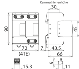
Maßbild DV M TN 255 FM
