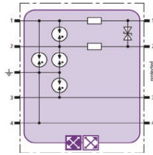
Prinzipialschaltbild BXT ML2 BD S EX 24
