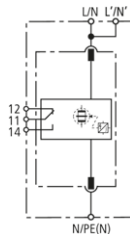
Prinzip Schaltbild DB M 1 150 FM
