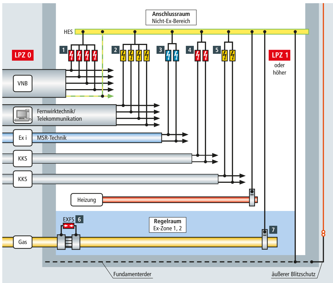
Bild 6 Blitzschutz-Potentialausgleich für eingeführte Leitungen
