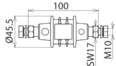
Maßbild EXFS 100
