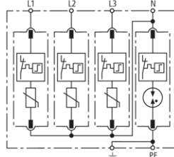
Principalschaltbild DG M TT 275
