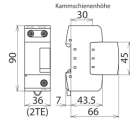
Maßbild DSE M 1 242
