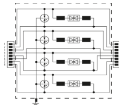
Prinzipialschaltbild DPA M CAT6 RJ45S 48
