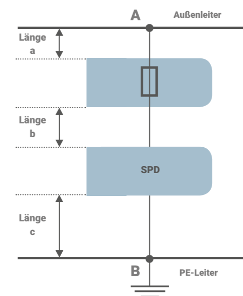
> Bild 9: Länge der Anschlussleitungen
