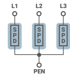
> Bild 6a: 3+0-Schaltung
