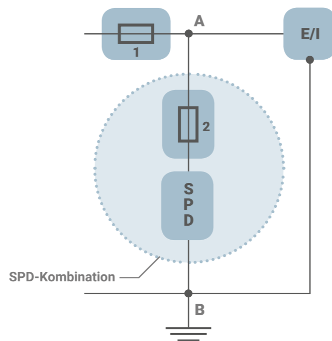
> Bild 8: SPD-Kombination
