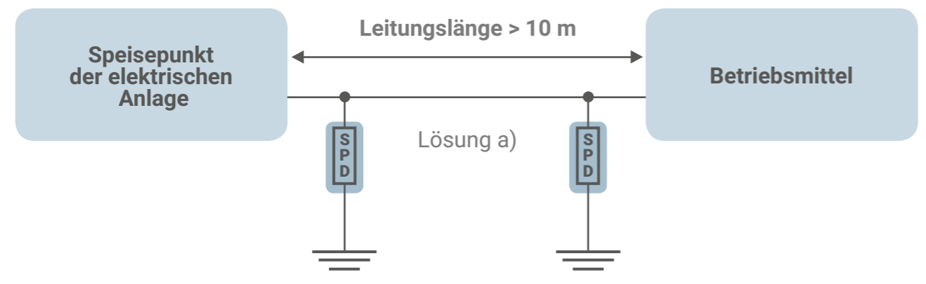
> Bild 5: Schutzbereich eines SPDs
