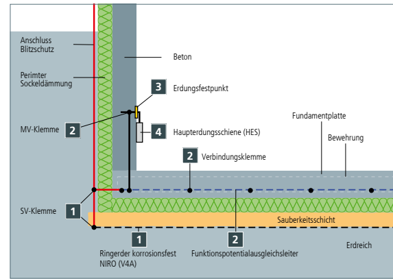
Anordnung des Fundamenterders bei einer geschlossenen Bodenplatte (vollisoliert) entsprechend DIN 18014
