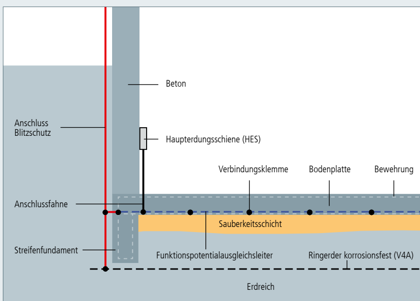
Bild 6: Anordnung des Fundamenterders bei bewehrter Bodenplatte und bewehrtem Streifenfundament entsprechend DIN 18014
