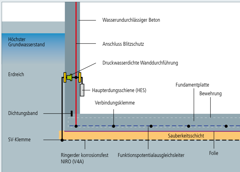
Bild 4: Anordnung eines Fundamenterders bei einer „Weißen Wanne“ entsprechend DIN18014
