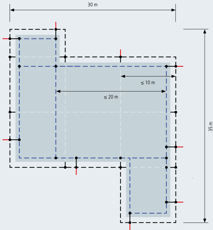
Bild 2: Fundamenterder in Maschenform bei einem größeren Gebäude
