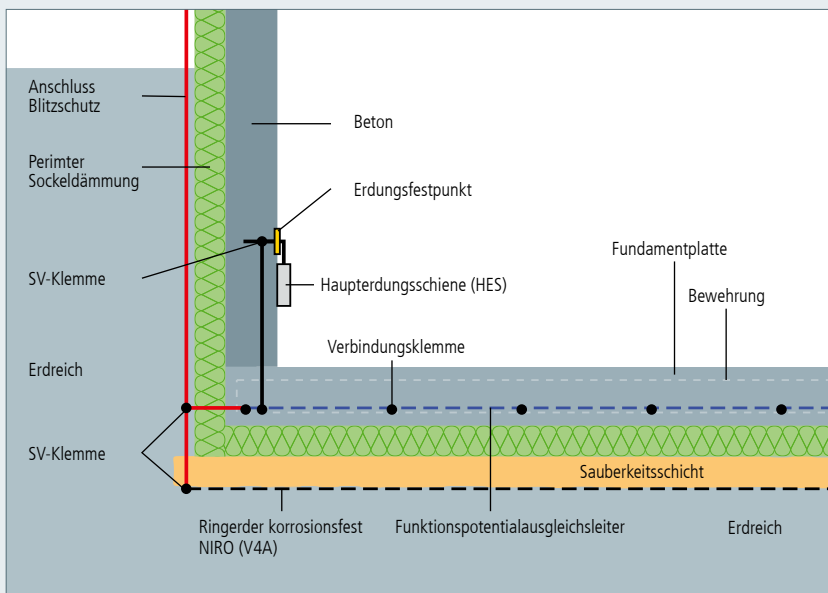
Bild 5: Anordnung des Fundamenterders bei einer geschlossenen Bodenplatte (vollisoliert) entsprechend DIN 18014
