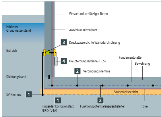
Anordnung eines Fundamenterders bei einer „Weißen Wanne“ entsprechend DIN18014
