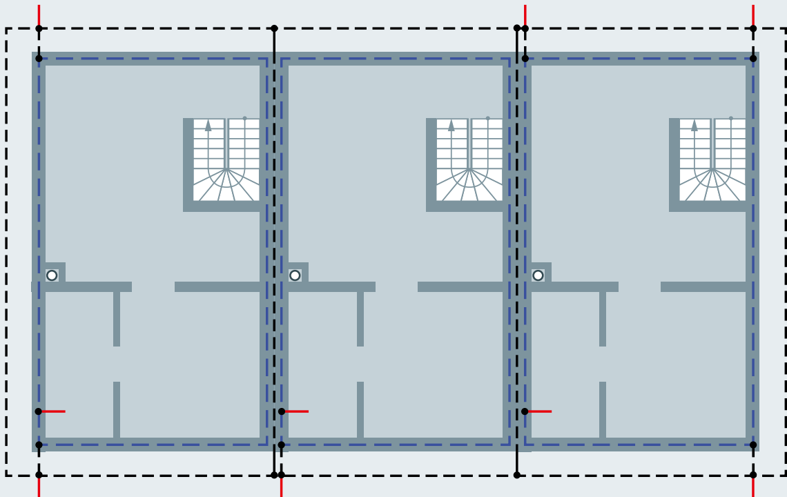
Bild 3: Fundamenterder bei Reihenhäusern
