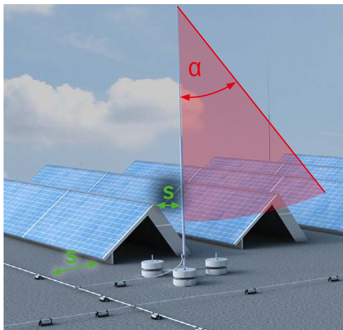
Einhaltung des Trennungsabstands „s“ und Ausbildung des Schutzbereichs für PV-Anlagen
