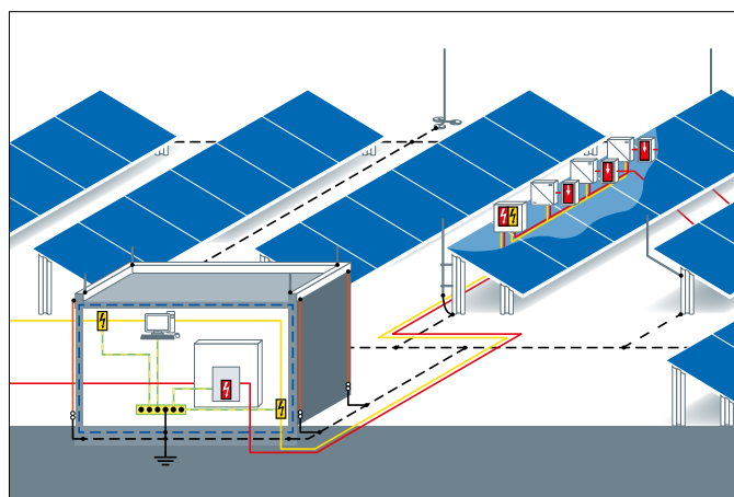
Solarpark mit Stringwechselrichter
