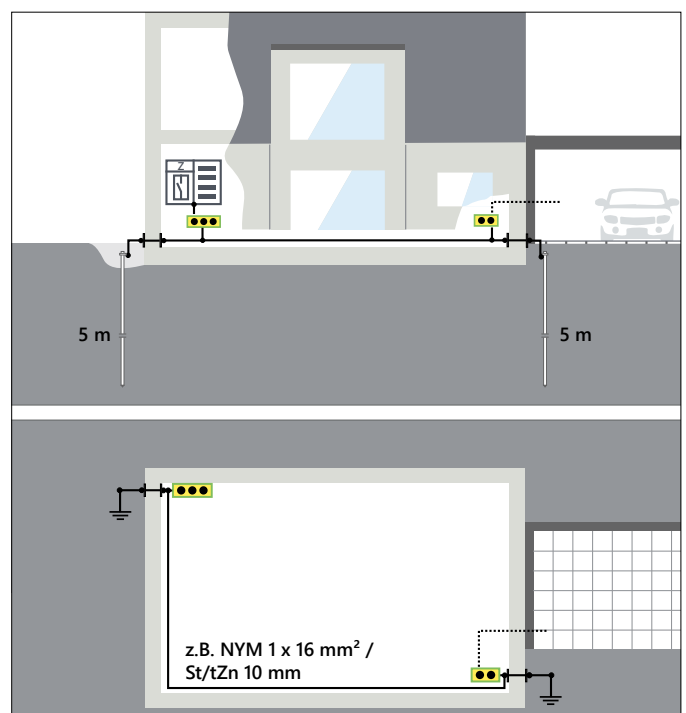
Nachrüstung einer Erdungsanlage mit zwei Tiefenerdern (5 m Länge) außerhalb und entsprechender Verbindungsleitung innerhalb des Gebäudes.
