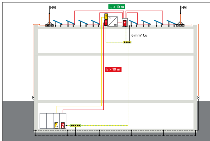
Gebäude mit HVI Blitzschutz: Trennungsabstand eingehalten (optimale Nutzung der vorhandenen Dachfläche für das PV-Systems)
