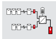
2 MPP / 2 String
