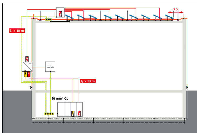
Gebäude mit äußerem Blitzschutzsystem: Trennungsabstand nicht eingehalten
