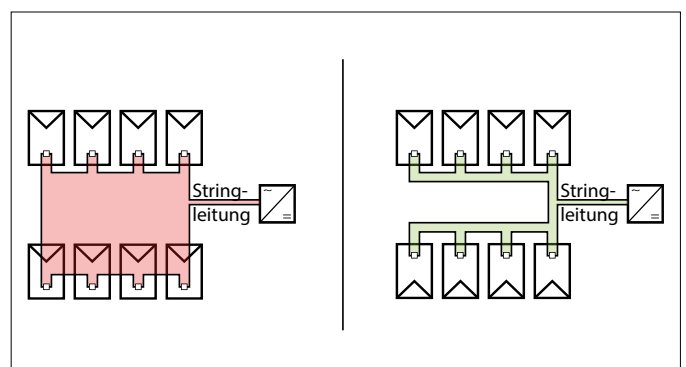
Große Koppelfläche
