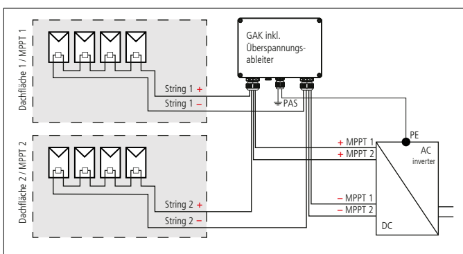
Anschlussbeispiel eines PV-Systems auf zwei Dachflächen (Ost-West-Ausrichtung)
