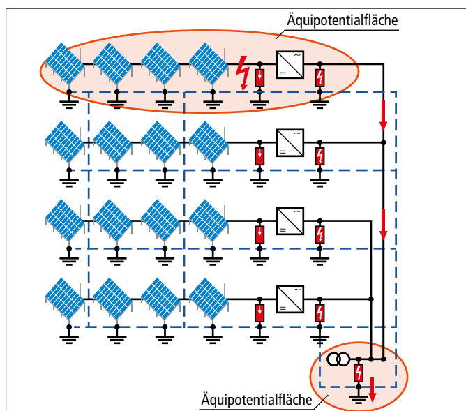
Vermashtes Erdungssystem
