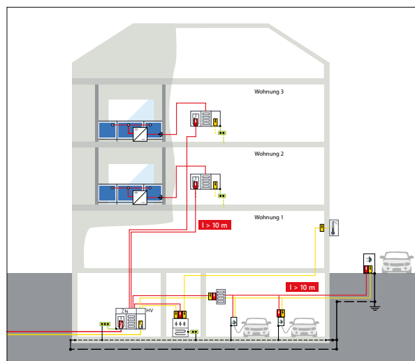
Gebäude ohne äußeres Blitzschutzsystem: Balkonkraftwerk
