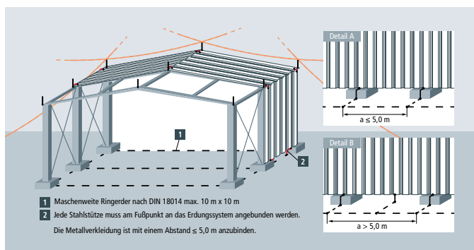
Einbindung der Stahlhalle in das Blitzschutzsystem
