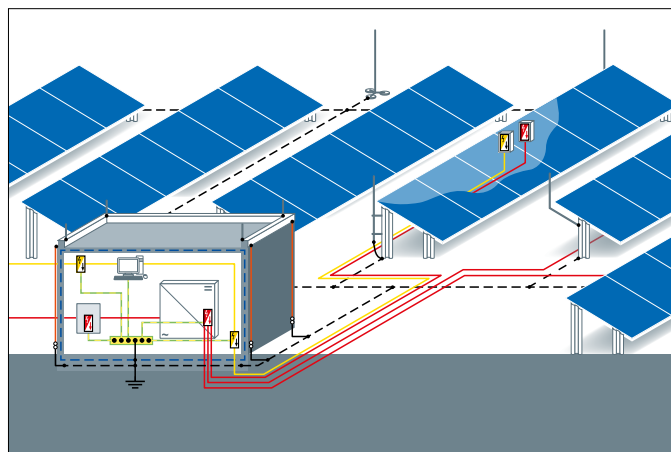
Solarpark mit Zentralwechselrichter
