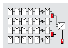
2 MPP / 2 String
