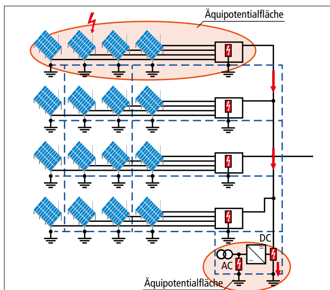
Vermaschtes Erdungssystem
