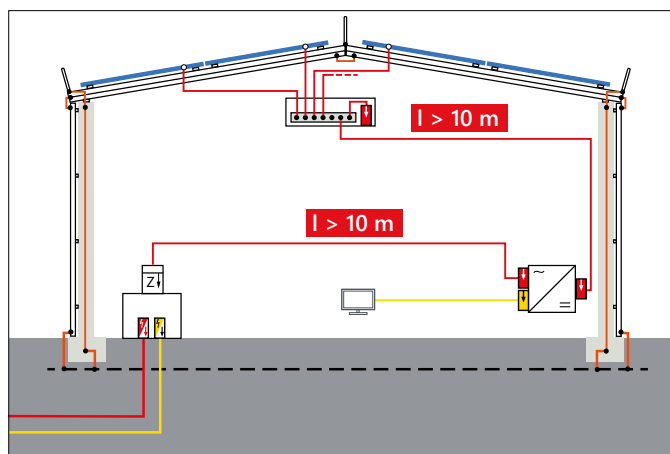
Gebäude mit äußerem Blitzschutzsystem: Metалldach
