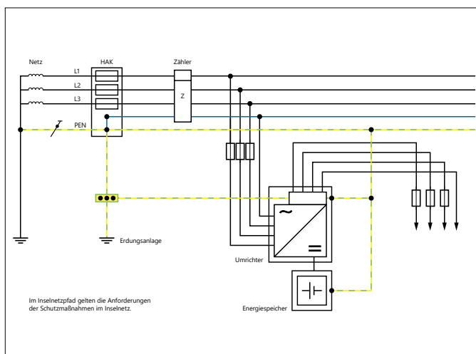
Auslegung einer funktionsfähigen Erdungsanlage bei Inselbetrieb einer PV-Anlage mit Batteriespeicheranwendung.
