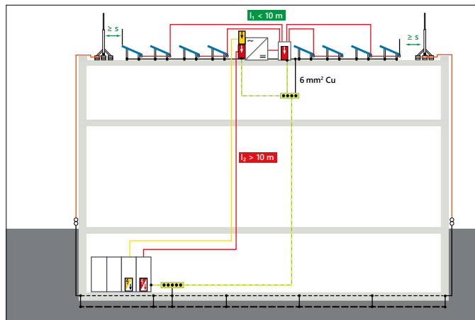
Gebäude mit konventionellem Blitzschutz: Trennungsabstand eingehalten
