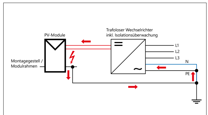
Isolationsfehler im DC-System bei trafolosen Wechselrichtern
