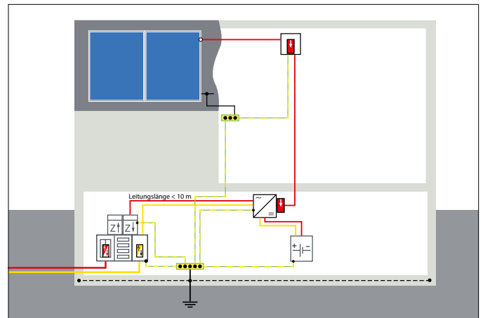
Wohngebäude ohne äußeres Blitzschutzsystem: Neubau
