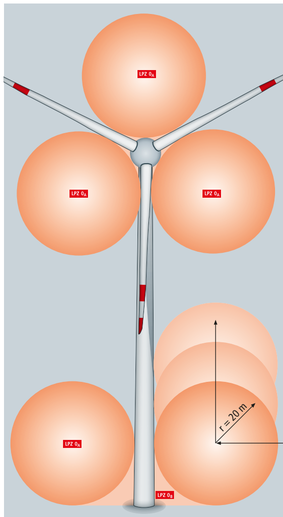
Bild 1 Blitzkugelverfahren
