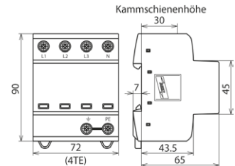
Maßbild DSH TT 255
