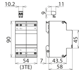
Maßbild BVT KKS ALD 75
