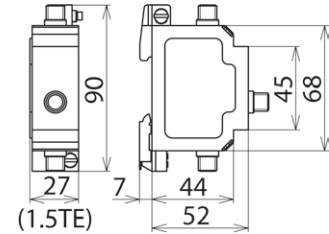
Maßbild DGA FF TV
