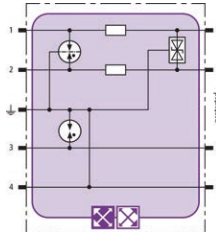
Prinzipialschaltbild BXT ML2 BE HFS 5
