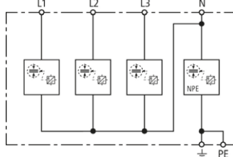
Prinzipialschaltbild DSH TT 255
