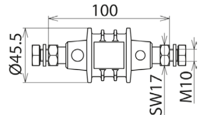
Maßbild EXFS 100
