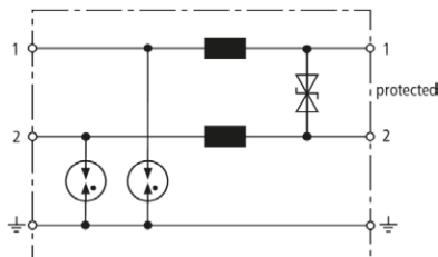
Prinzipschaltbild BVT ALD 36
