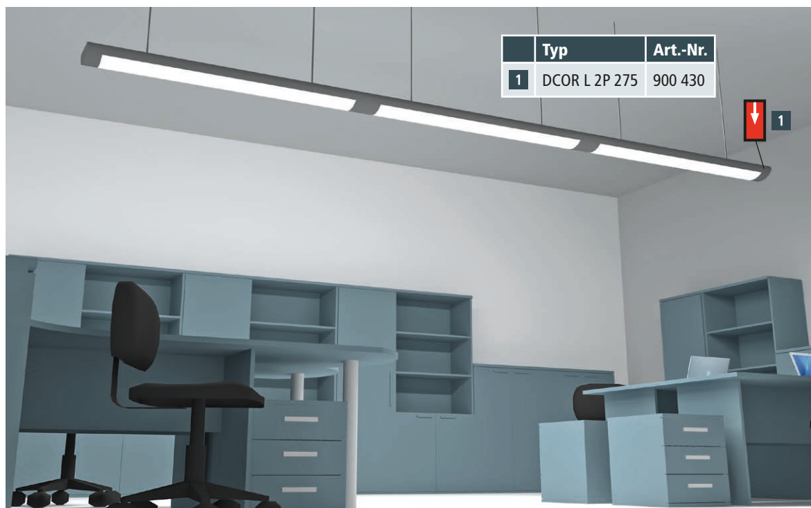
Bild 1 Überspannungs-Ableiter Typ 3 in Büroraumleuchten
