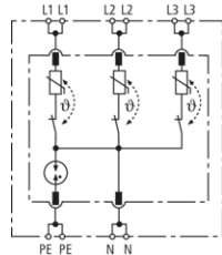
Prinzipialschaltbild DR M 4P 255
