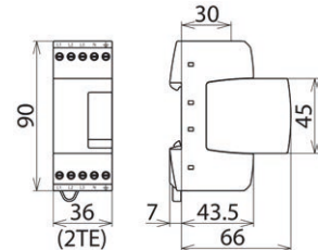
Maßbild DR M 4P 255
