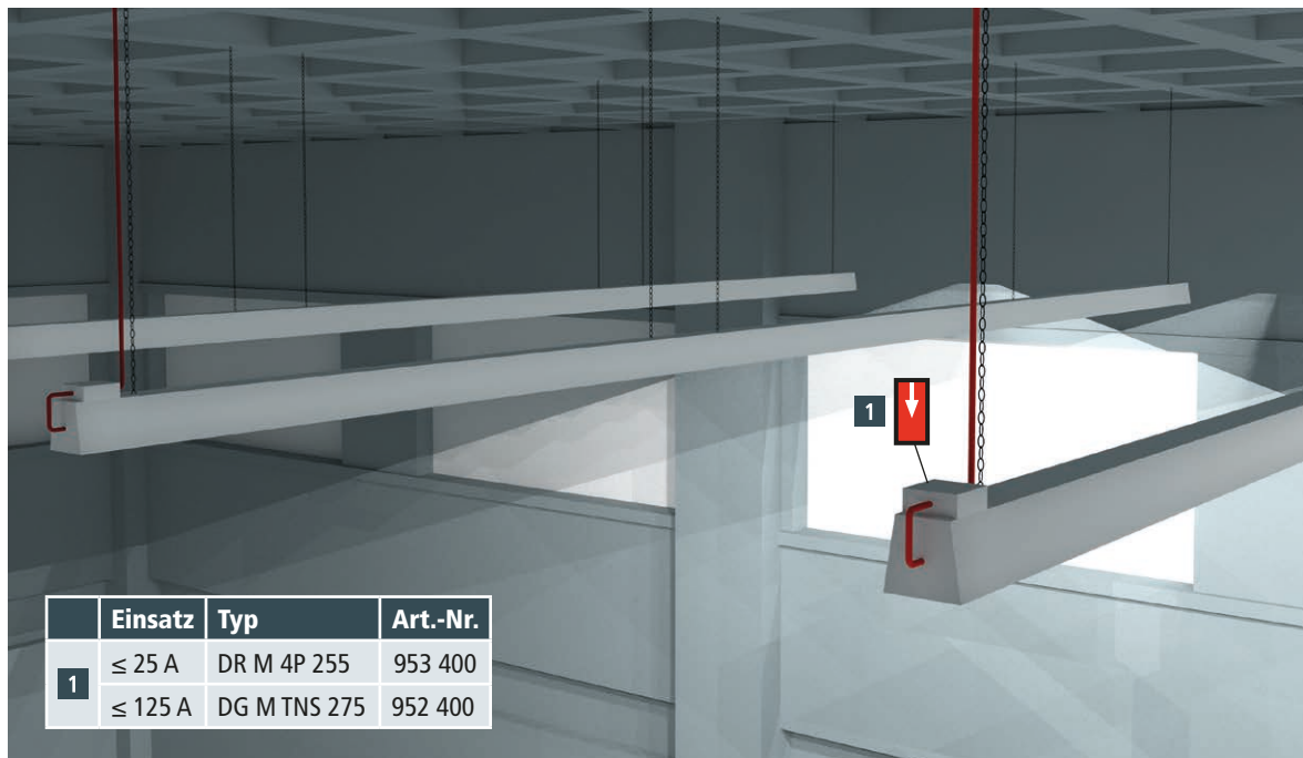
Bild 2 Überspannungs-Ableiter Typ 3 bzw. Typ 2 im AP-Gehäuse auf der Lichtbandleuchten-Tragschiene
