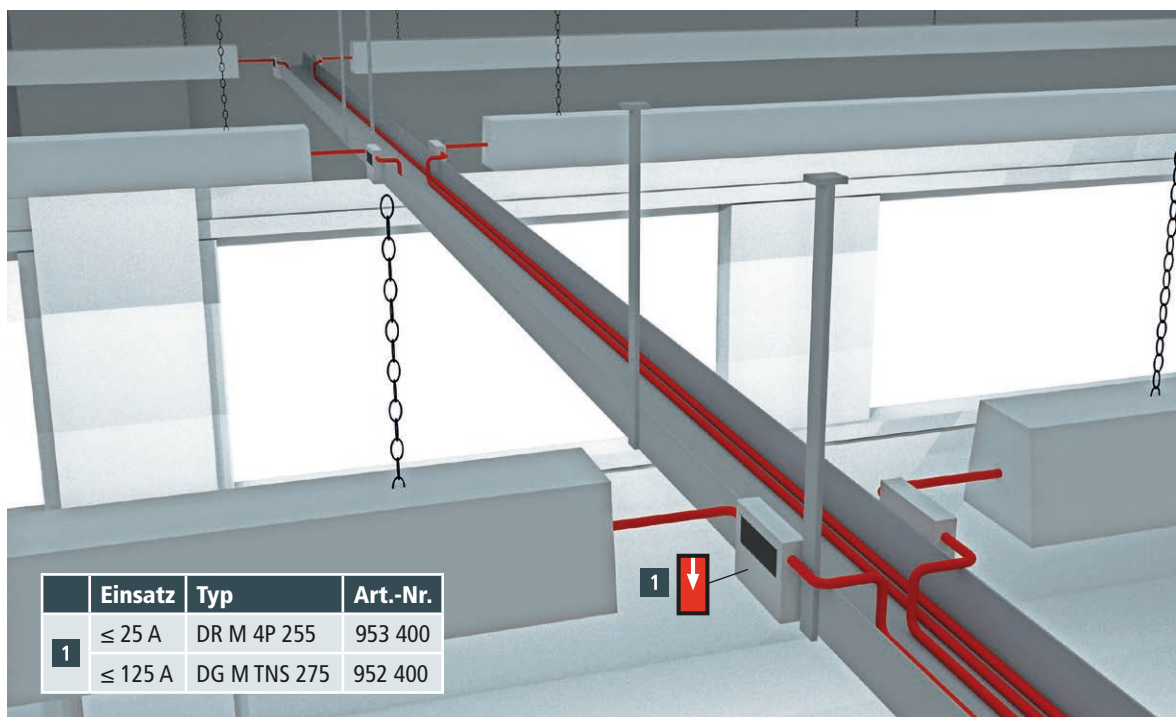
Bild 3 Überspannungs-Ableiter Typ 3 bzw. Typ 2 im AP-Gehäuse auf der Kabelrinne
