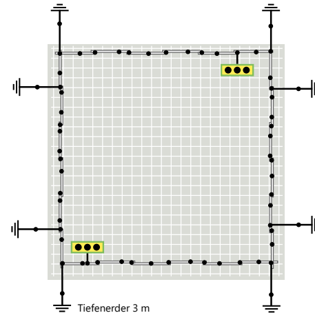
Ausführung 8 Tiefenerder mit je 3 m
