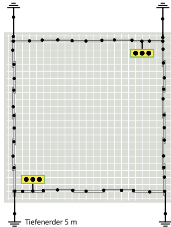
Ausführung 4 Tiefenerder mit je 5 m
