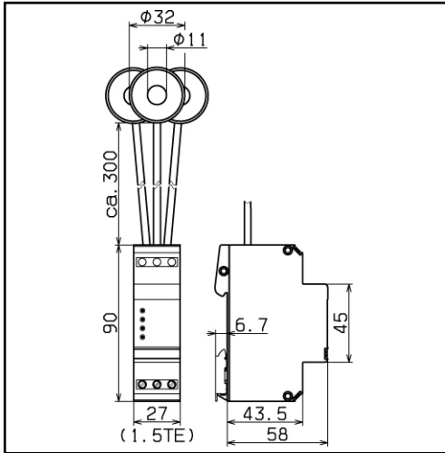
Maßbild DISO 3
