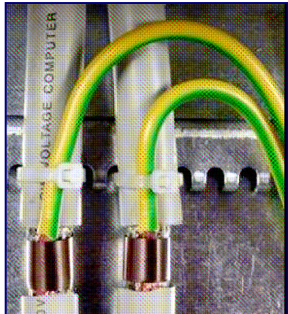
Bild 3: Schirmanschlusssystem SA KRF
