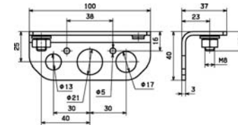
Befestigungswinkel aus Edelstahl mit 3 Montagelöchern Art.-Nr. 106 329 Geeignet für 3 verschiedene DEHNgate Art.-Nr. 1 x 929 042 + 1 x 929 057 + 1 x (929 043, 929 044, 929 045 oder 929 059) Stainless steel angled fixing plate with 3 mounting holes Part No. 106 329 For 3 different DEHNgate types Part Nos. 1 x 929 042 + 1 x 929 057 + 1 x (929 043, 929 044, 929 045 or 929 059)
