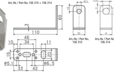
Befestigungswinkel aus Edelstahl Art.-Nr. 106 310 Geeignet für DEHNgate Art.-Nr. 929 045 - 929 048 und 929 446 Art.-Nr. 106 314 Geeignet für DEHNgate Art.-Nr. 929 043 - 929 045 Stainless steel angled fixing plate, Part No. 106 310 For DEHNgate Part Nos. 929 045 - 929 048 and 929 446 Part No. 106 314 For DEHNgate Part Nos. 929 043 - 929 045
