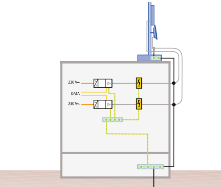
Potentialausgleichsleiter \geq 10 \text{ mm}^2 \text{ Cu} Equipotential bonding conductor \geq 10 \text{ mm}^2 \text{ Cu}
