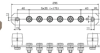
Potentialausgleichsschiene aus Edelstahl, Montagelochabstand 35 mm Art.-Nr. 472 209 Geeignet für 3 x DEHNgate Art.-Nr. 929 045 - 929 048 und 929 446 Stainless steel equipotential bonding bar, distance between mounting holes 35 mm Part No. 472 209 For 3 x DEHNgate Part Nos. 929 045 - 929 048 and 929 446
