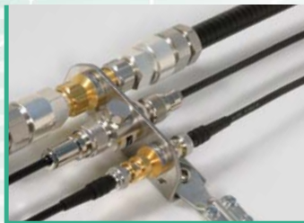
Durchsteckmontage von DEHNgates Art.-Nr. 929 042, 929 044 und 929 057 im Befestigungswinkel Art.-Nr. 106 329 und zusätzlich Erdungskabel Art.-Nr. 416 411 Through-hole mounting of DEHNgate Part Nos. 929 042, 929 044 and 929 057 in the angled fixing plate Part No. 106 329 and additional earthing cable Part No. 416 411
