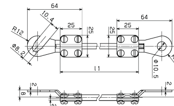
Hochflexible Erdungsleitung (1 m) mit Kabelschuhen, 100 kA (10/350 µs) Art.-Nr. 416 411 Geeignet für die Kombination mit Art.-Nr. 106 310, 106 329 und 472 209 Highly flexible earthing conductor (1 m) with cable lugs, 100 kA (10/350 µs) Part No. 416 411 For combination with Part Nos. 106 310, 106 329 and 472 209
