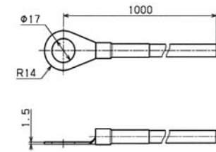
Kabelschuh mit Erdungskabel Art.-Nr. 929 096 Geeignet für DEHNgate Art.-Nr. 929 043, 929 044 und 929 045 Cable lug with earthing cable Part No. 929 096 For DEHNgate Part Nos. 929 043, 929 044 and 929 045
