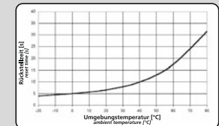
Rückstellzeit, nach der das Gaskapselsystem bei gegebener Umgebungstemperatur in den normalen Betriebszustand zurückkehrt. Reset time after which the gas capsule system returns to its normal operating state at a given ambient temperature.
