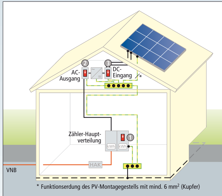
Bild 1.3 Überspannungsschutz-Konzept für eine PV-Anlage auf einem Gebäude ohne Äußeren Blitzschutz
